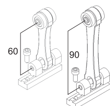
Polea corredera c/prolongación
