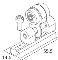
Polea corredera
