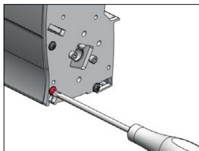
Detalle del montaje para máquina
