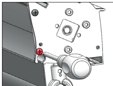
Detalle del montaje del perfil registro
