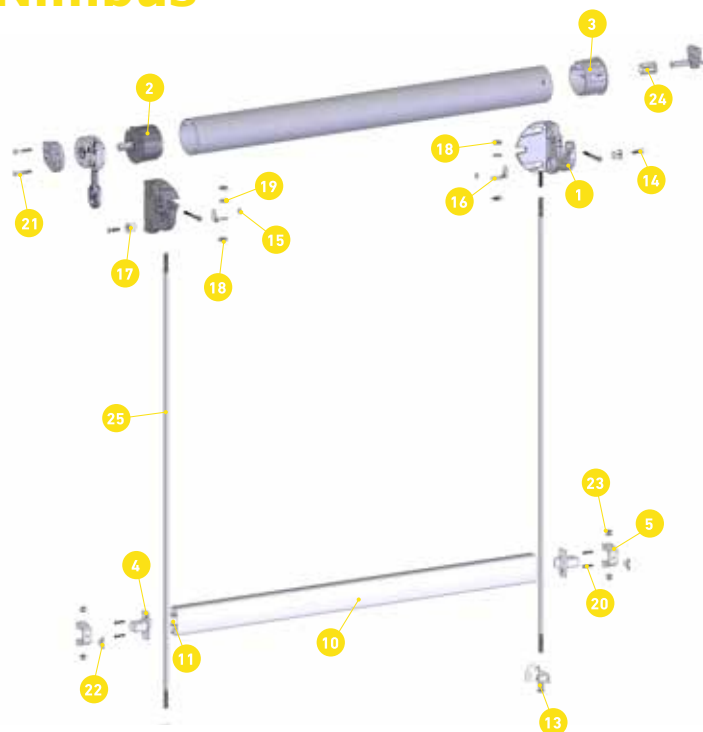
E Esquema Screen Nimbus varilla Ø10 con máquina.
