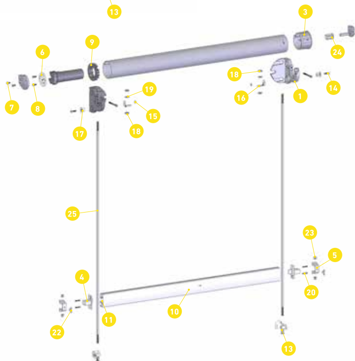
F Schéma Store Vertical Nimbus avec tringle Ø10, motorisé.
