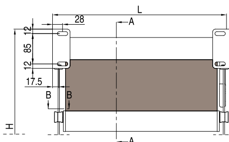
supporto a parete - wall bracket
