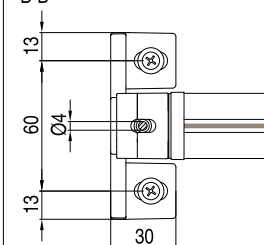
piedino a pavimento - floor bracket B-B
