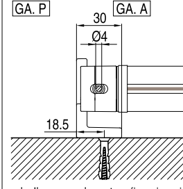
piedino a pavimento - floor bracket B-B
