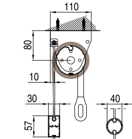
GA Posteriore - GA back A-A
